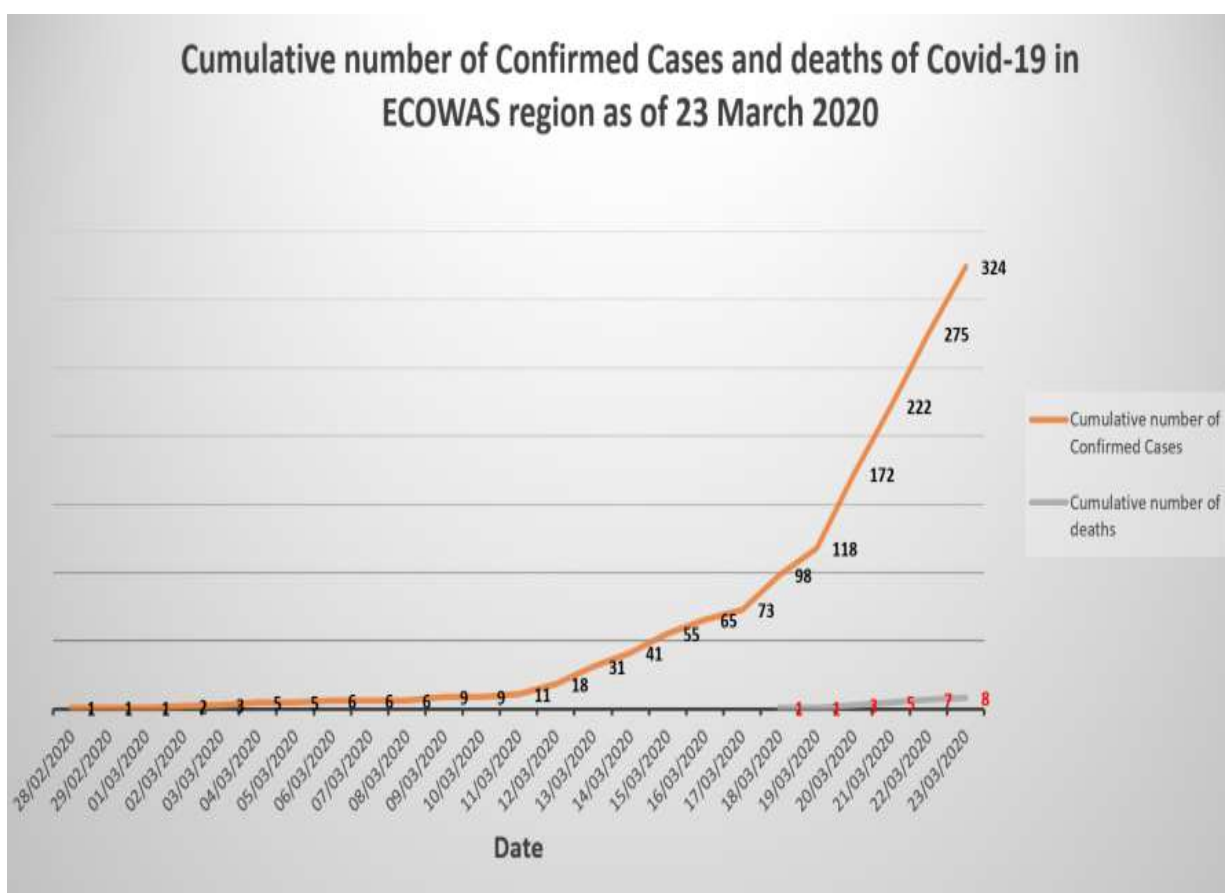
Fig 1: Nombre cumulé des cas confirmés et des décès de Covid-19 dans l'espace CEDEAO au 23/03/20 / Cumulative Number of Confirmed Cases and deaths of Covid-19 in ECOWAS region as of 23 March 2020.
